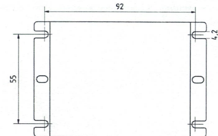
Abbildung 2: Abmessungen der Anschraubpunkte des Gehäuses
